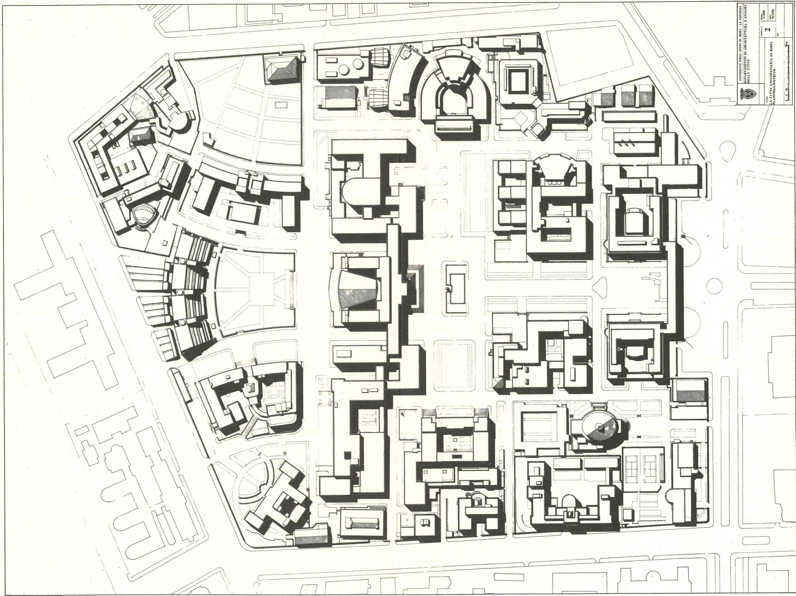
Planivolumetrico della Città Universitaria, 1985.
